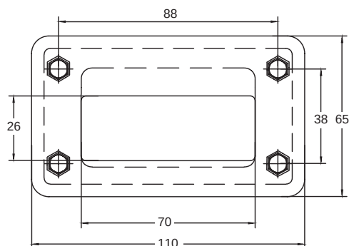
內牙固定型 In Stationary type HP-008-2
