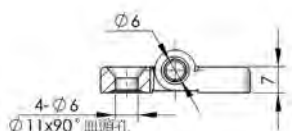
圓頭孔型 Countersunk
