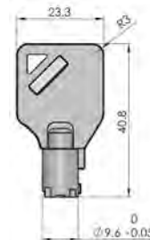
鑰匙 KEY
