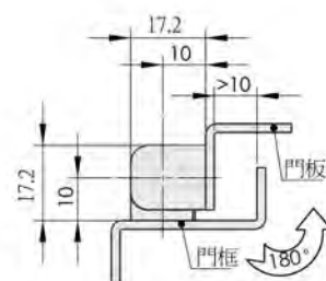
CL-203-3 同軸鉸鏈
