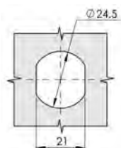
開孔尺寸 Cut Out
