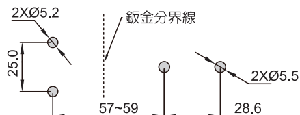
水平式安裝開孔尺寸
