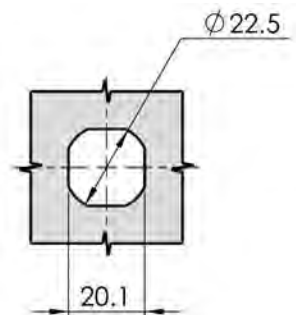
開孔尺寸 Cut Out
