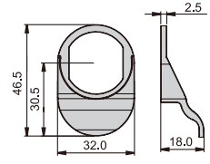
取手
