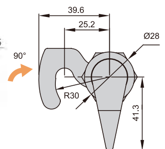
標準擋片
