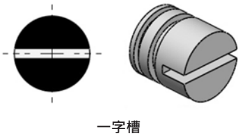
一字槽
