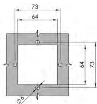
開孔尺寸 Cut Out
