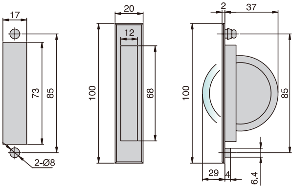
開孔尺寸 Cut Out
