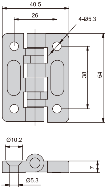
CL-209-2R 皿頭孔型 Countersunk Type
