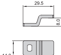
標準擋片 (Standard Cam Type)
