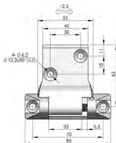
安裝示意圖
