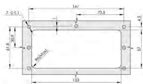
開孔尺寸 Cut Out
