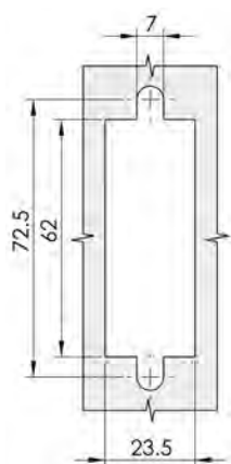
開孔尺寸 Cut Out
