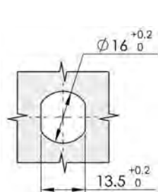
開孔尺寸 Cut Out
