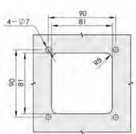
開孔尺寸 Cut Out
