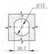
開孔尺寸 Cut Out
