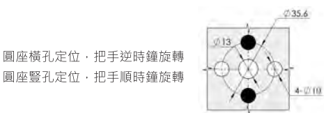
開孔尺寸 Cut Out
