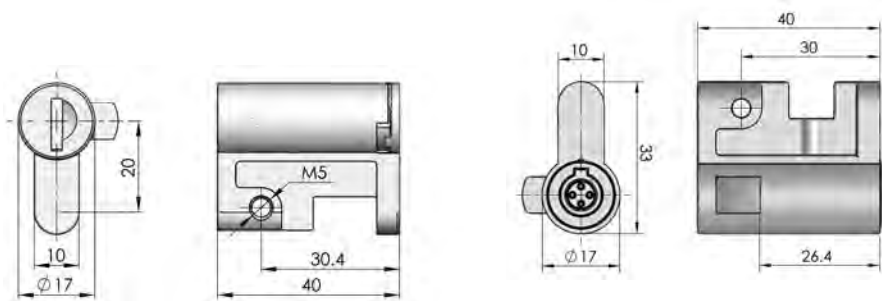
標準鎖芯 Standard Lock Cylinder
