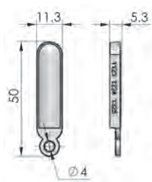
磁鐵 KEY
