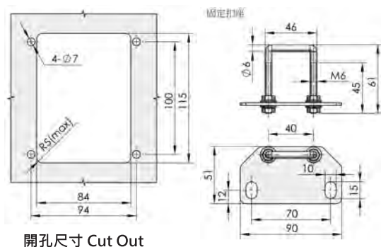
開孔尺寸 Cut Out
