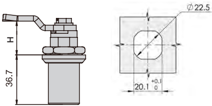
開孔尺寸 Cut Out
