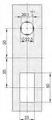
開孔尺寸 Cut Out
