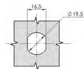
開孔尺寸 Cut Out
