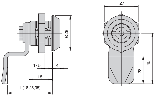
8X8mm 四角型
