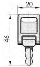
鑰匙 KEY
