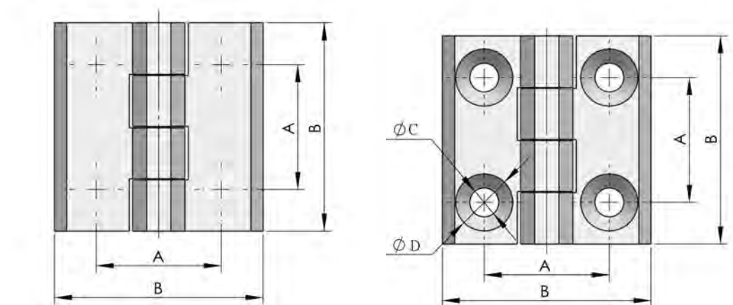
螺柱型 Thread-stud
