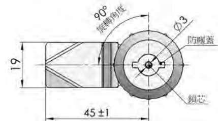
擋片可選 DS1B45 系列 (外定位)
