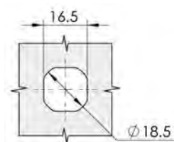
開孔尺寸 Cut Out
