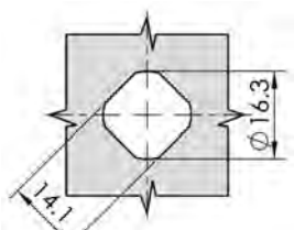
開孔尺寸 Cut Out
