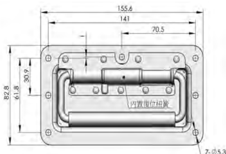
開孔尺寸 Cut Out
