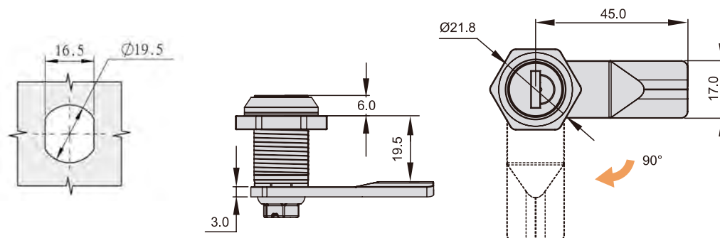
開孔尺寸 Cut Out
