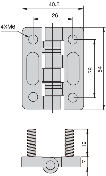
CL-209-1R 螺柱型 Thread-stud Type
