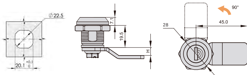
開孔尺寸 Cut Out
