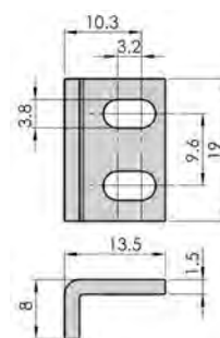
固定扣
