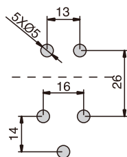
開孔尺寸 Cut Out
