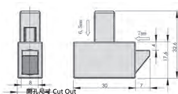
開孔尺寸 Cut Out
