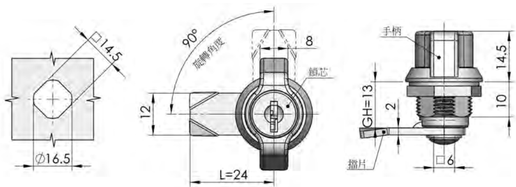
開孔尺寸 Cut Out
