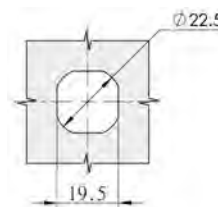
開孔尺寸 Cut Out
