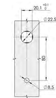
開孔尺寸 Cut Out
