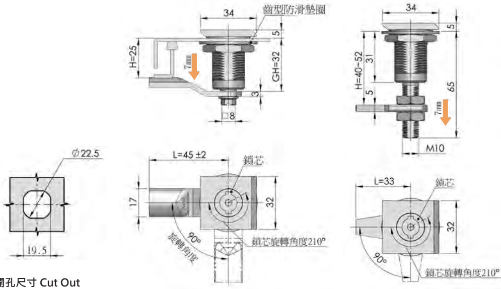
可調間距型 (Adjustable grip)
