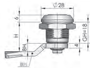
擋片可選 S1B45 系列
