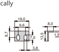
固定扣
