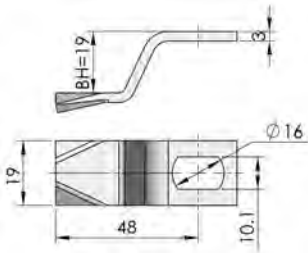
擋片
