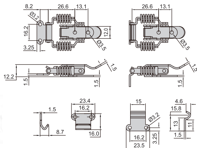
TS-33B 垂直安裝座
