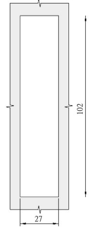
開孔尺寸 Cut Out
