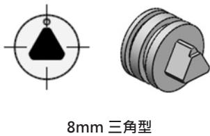
8mm 三角型
