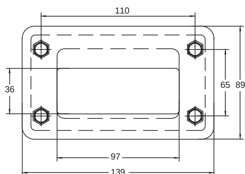
內牙固定型 In Stationary type HP-009-2
