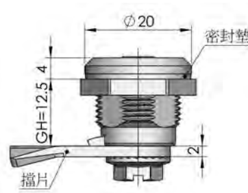
MS-845-1 (□ 6x6 四方型)
