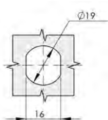
開孔尺寸 Cut Out
