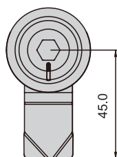
開孔尺寸 Cut Out
