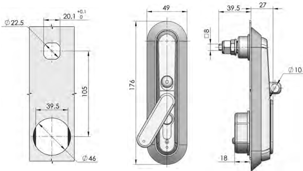
開孔尺寸 Cut Out
