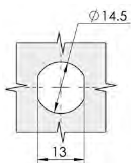
開孔尺寸 Cut Out
