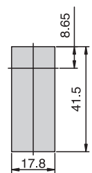
開孔尺寸 Cut Out
