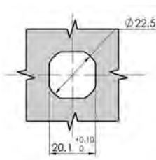
開孔尺寸 Cut Out
