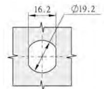
開孔尺寸 Cut Out
