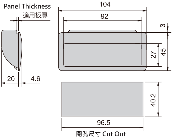
開孔尺寸 Cut Out
