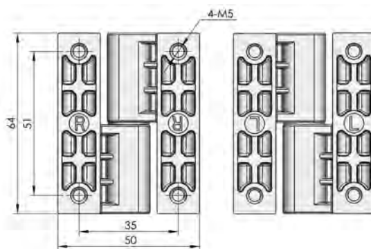
右開門
