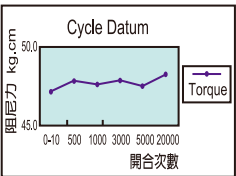
開合次數與扭力變化圖
